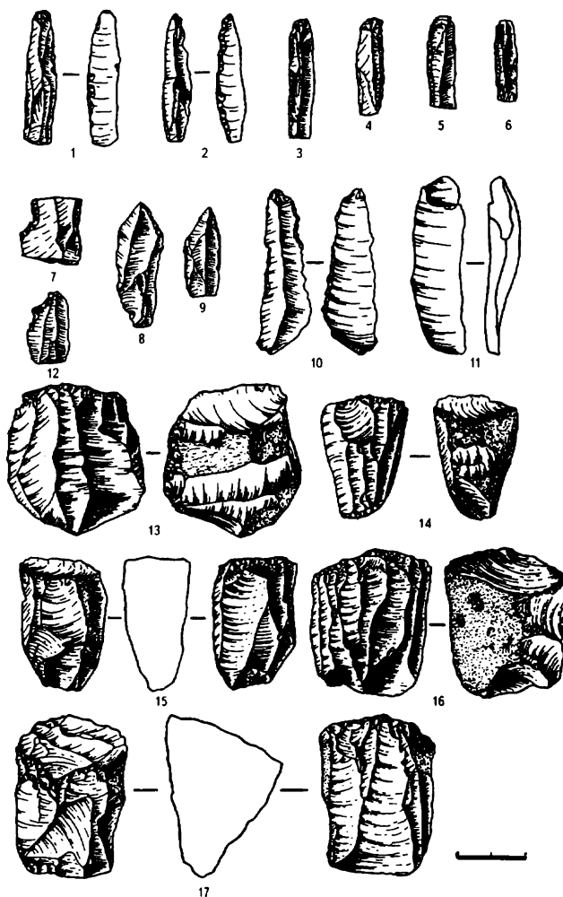
Рис. 3. Второй хозяйственно-бытовой комплекс: 1-6 – пластинки с притупленным краем; 7, 12 – скребели; 8-9 – клинки-наконечники; 10 – пилка (орудие с зубчатым краем); 11 – пластинка с подтеской ударного бугорка; 13-17 – нуклеусы.
