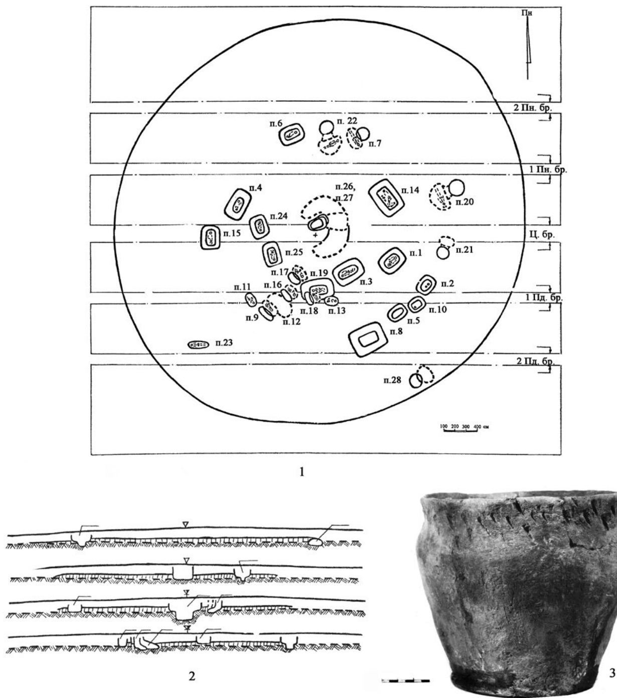
Рис. 6. Загальний план кургану №2 та зрубний горщик з насипу.
